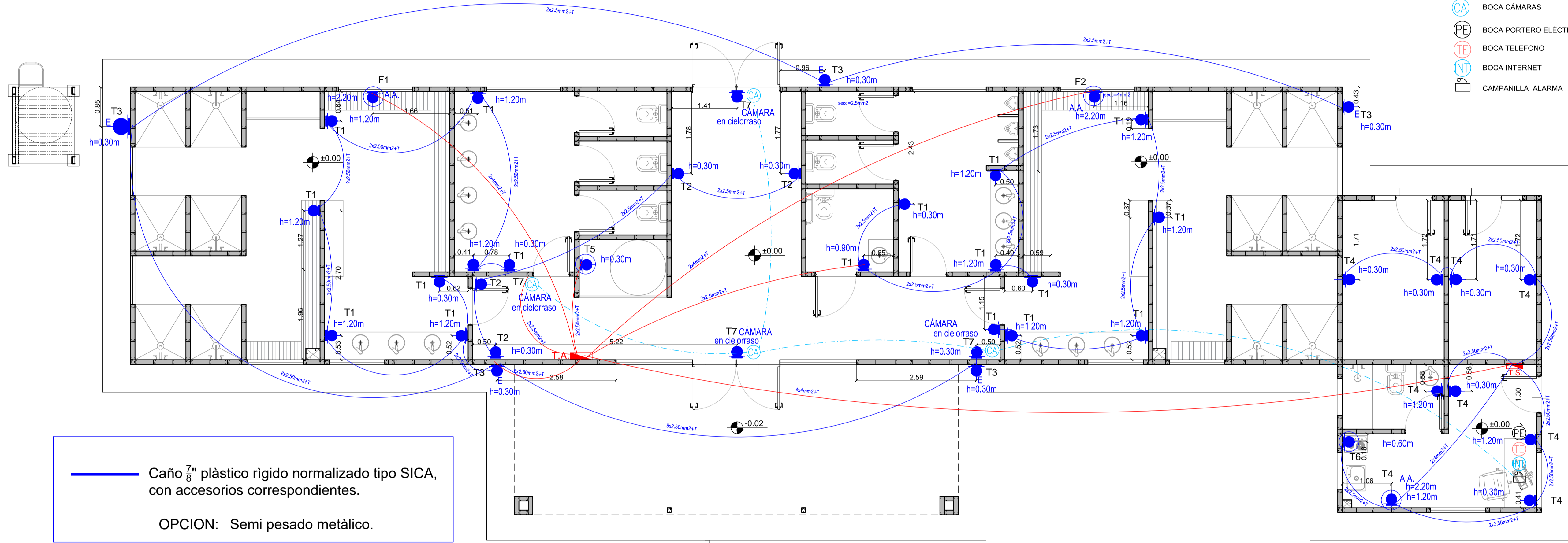
PLANTA GENERAL
