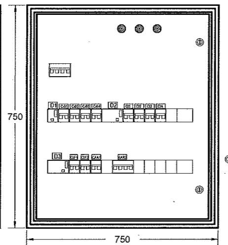
VISTA FRONTAL SIN PUERTA
